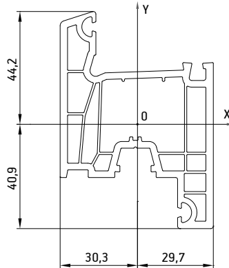
002 Створка
