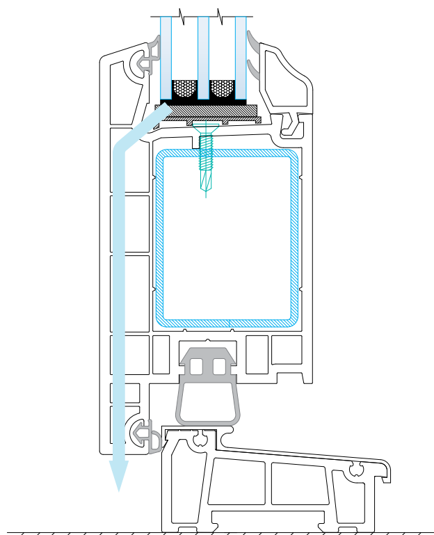
Рис.3в Типовые схемы вентиляции дверной створки
