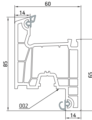
Створка 4-камерная 002
