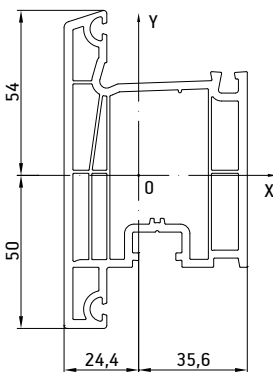
007 Дверная створка
