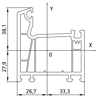
001 Рама
