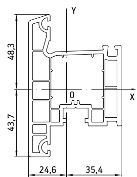
056 Дверная створка
